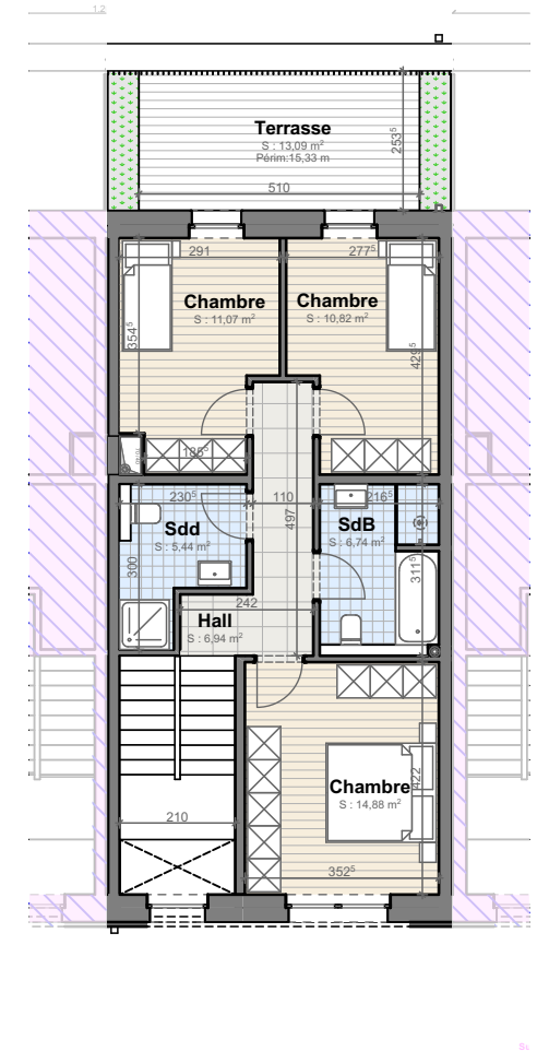
Etage +1
