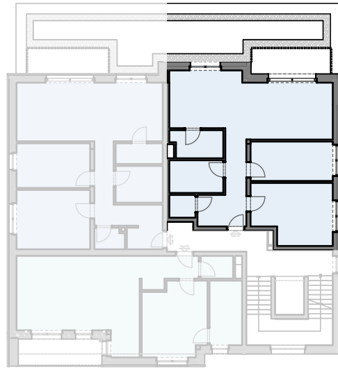
1er étage
